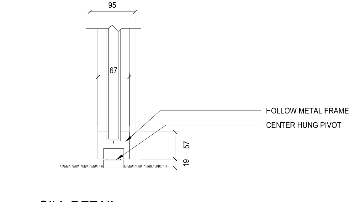
47 SILL DETAIL PIVOT DOOR 1/5
