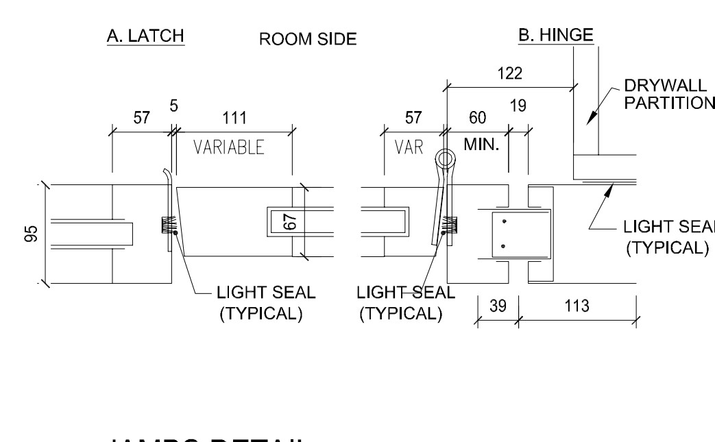
53 JAMBS DETAIL HINGED DOOR 1/5
