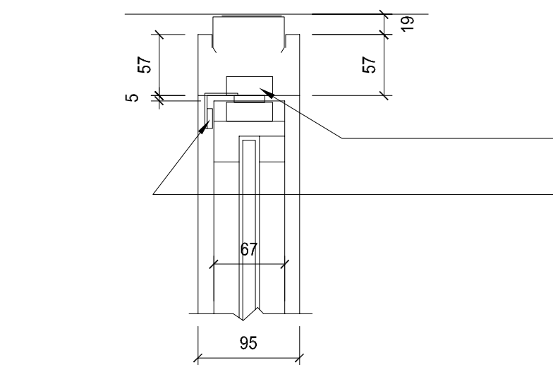
46 HEAD DETAIL PIVOT DOOR 1/5
