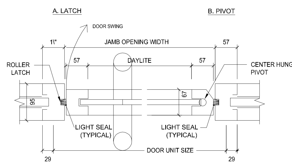
52 JAMBS DETAIL CENTER HUNG PIVOT DOOR 1/5
