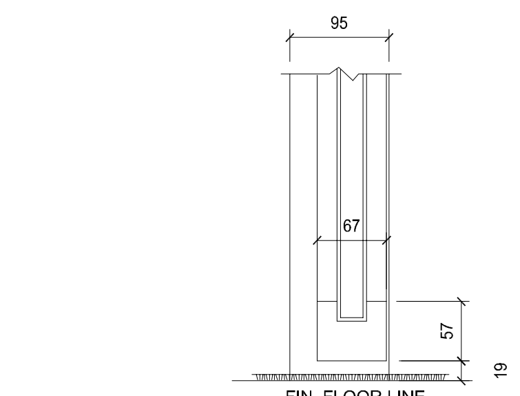
43 SILL DETAIL SLIDING DOOR 1/5
