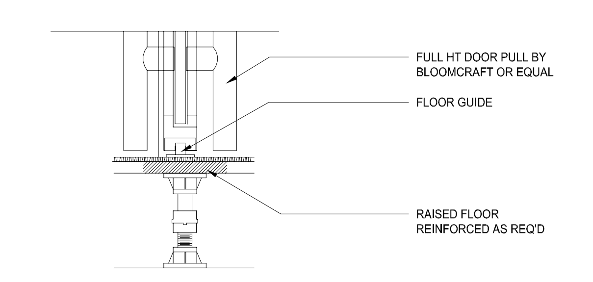
49 SILL DETAIL SLIDING DOOR 1/5
